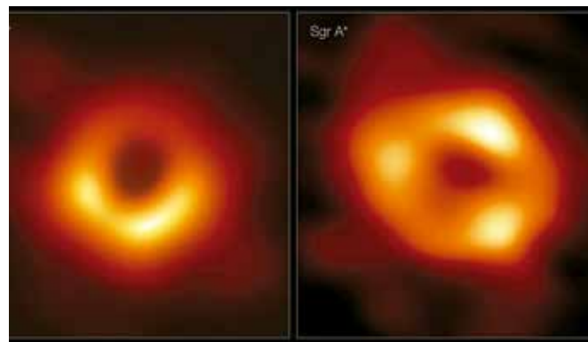
Foto: DPA Una imagen compuesta muestra un agujero negro en el centro de la galaxia gigante Messier 87.
